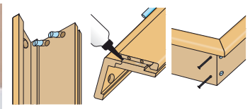
patentierte Zargenkonstruktion (GMF)
